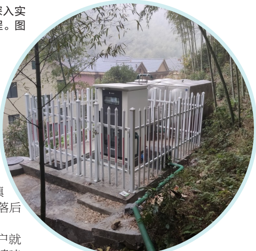
萧南山片高海拔区域泵站运维管理智慧化提升。图为河上镇大坞朱村泵站。
