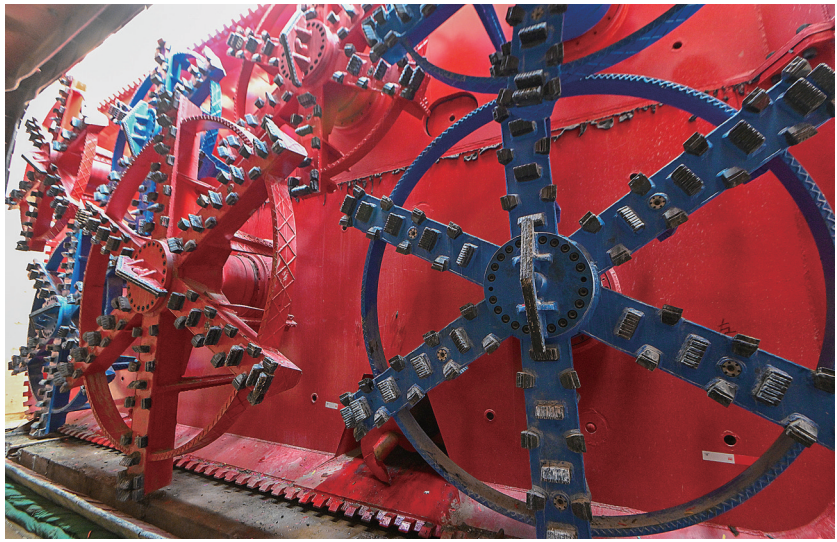
矩形顶管机始发。 记者 范方斌 摄
